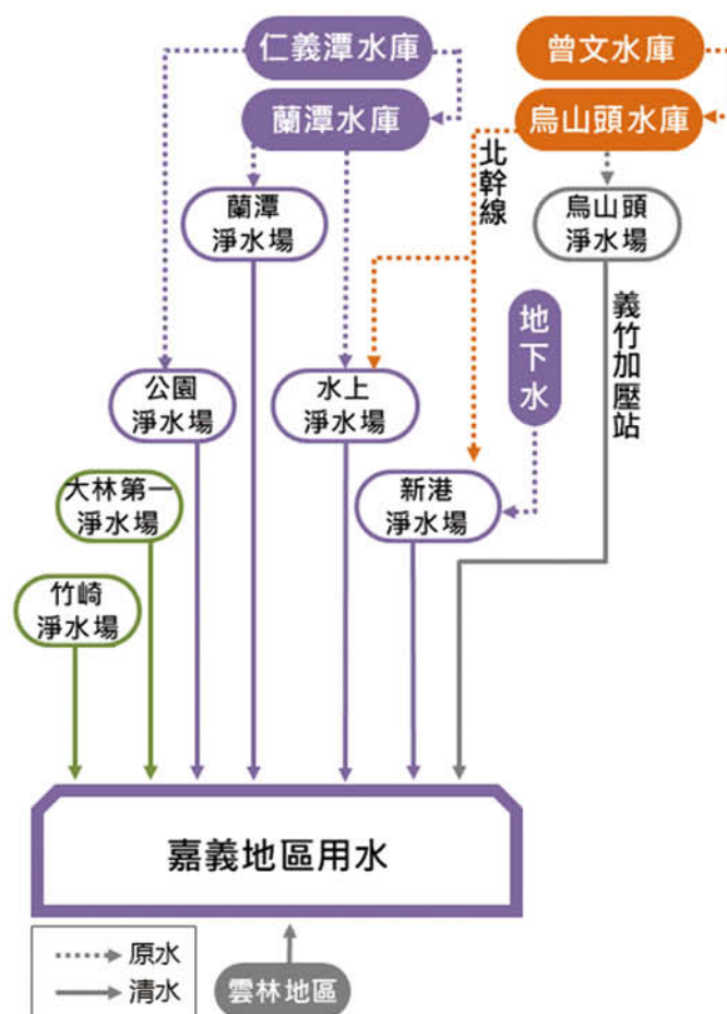
嘉義地區自來水水源供需圖
